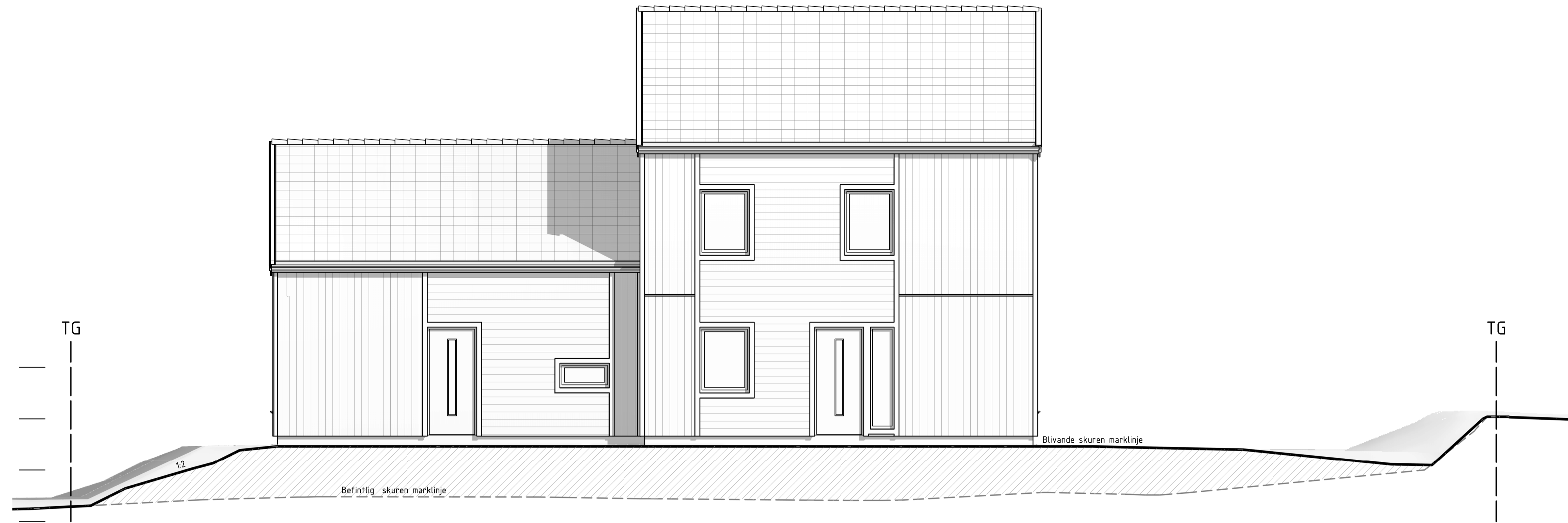
FASAD A 1 : 50 Fasadelevation mot norr
