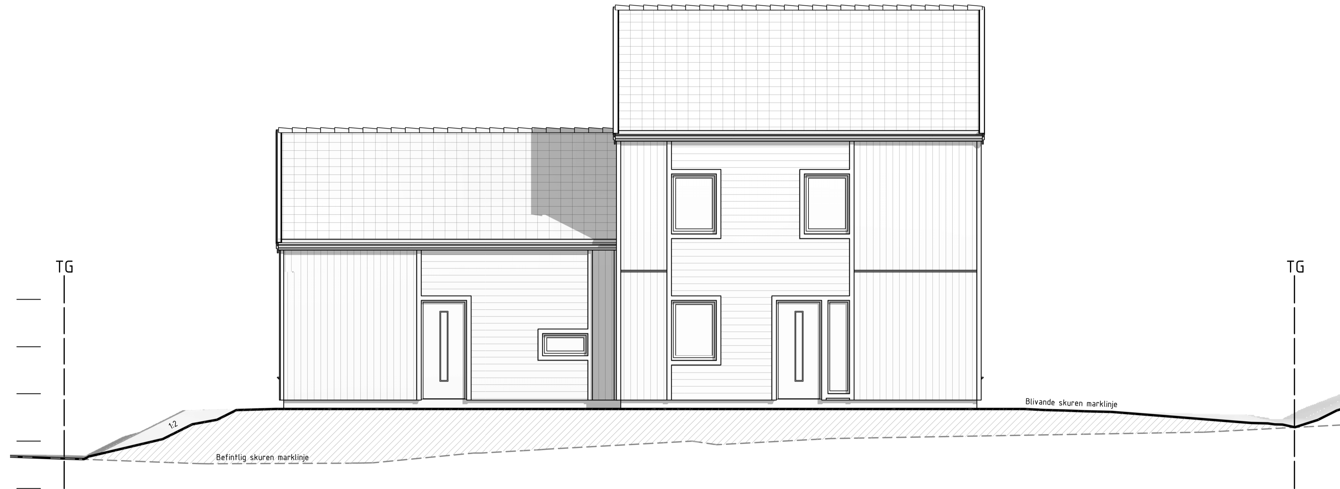
FASAD A 1 : 50 Fasadelevation mot norr
