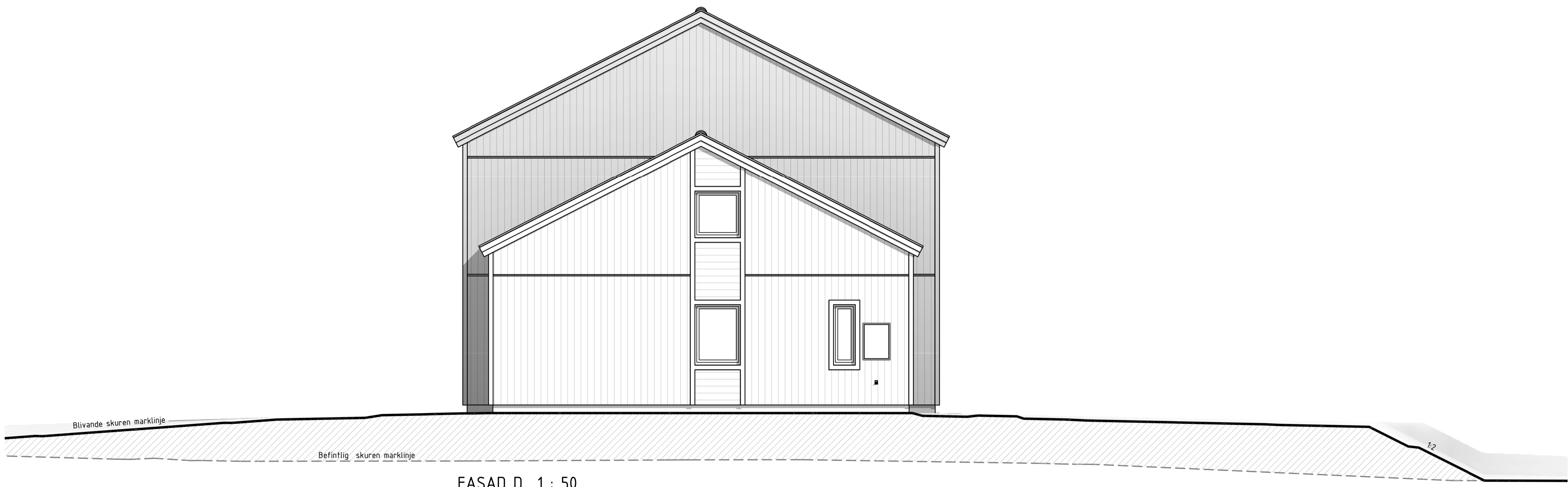
FASAD D 1 : 50 Fasadelevation mot öst
