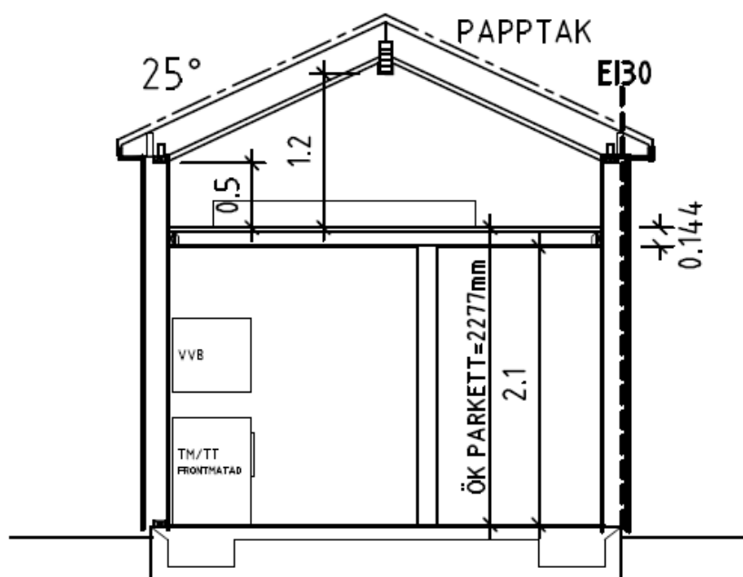
SEKTION A - A
