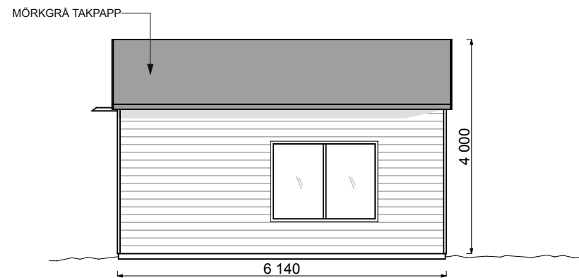
FASAD MOT ÖST
