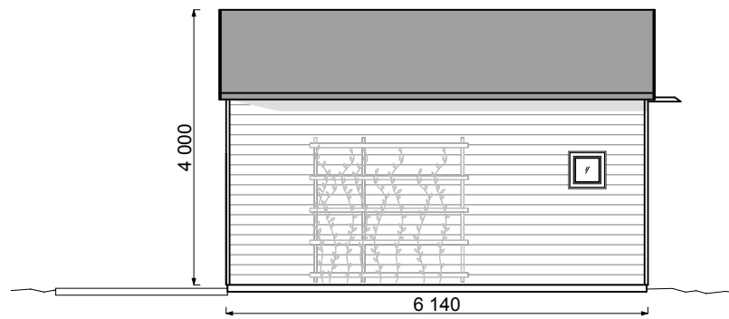
FASAD MOT VÄST
