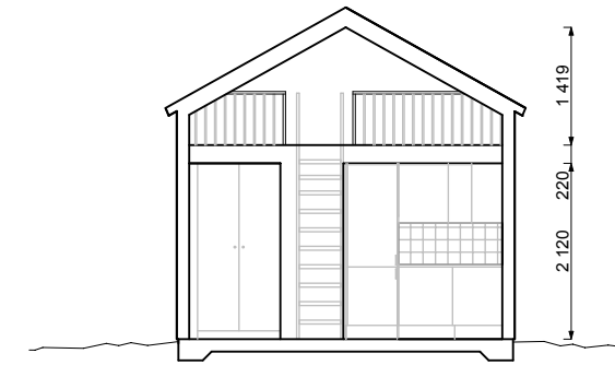
SEKTION A-A
